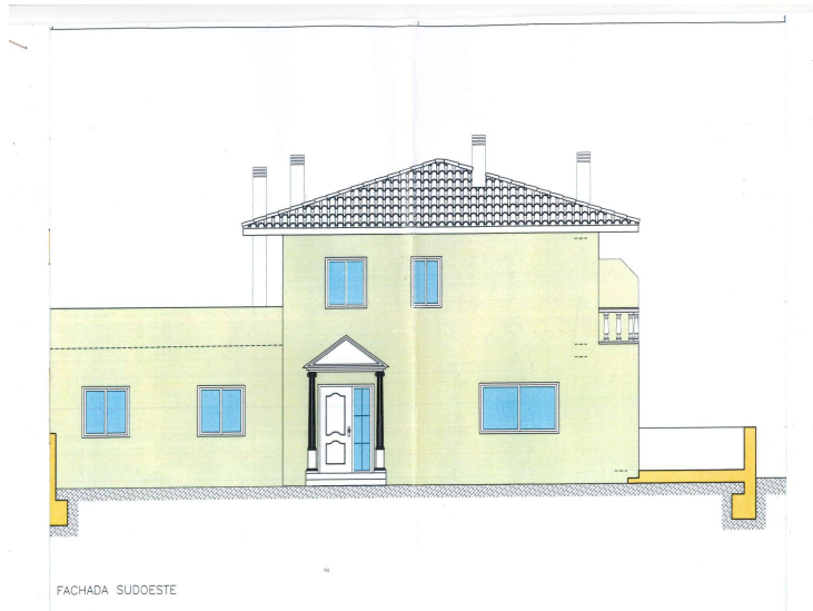
FACHADA SUDOESTE
