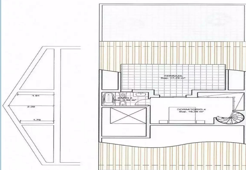
PLANTA BAJOCUBIERTA E: 1/100
